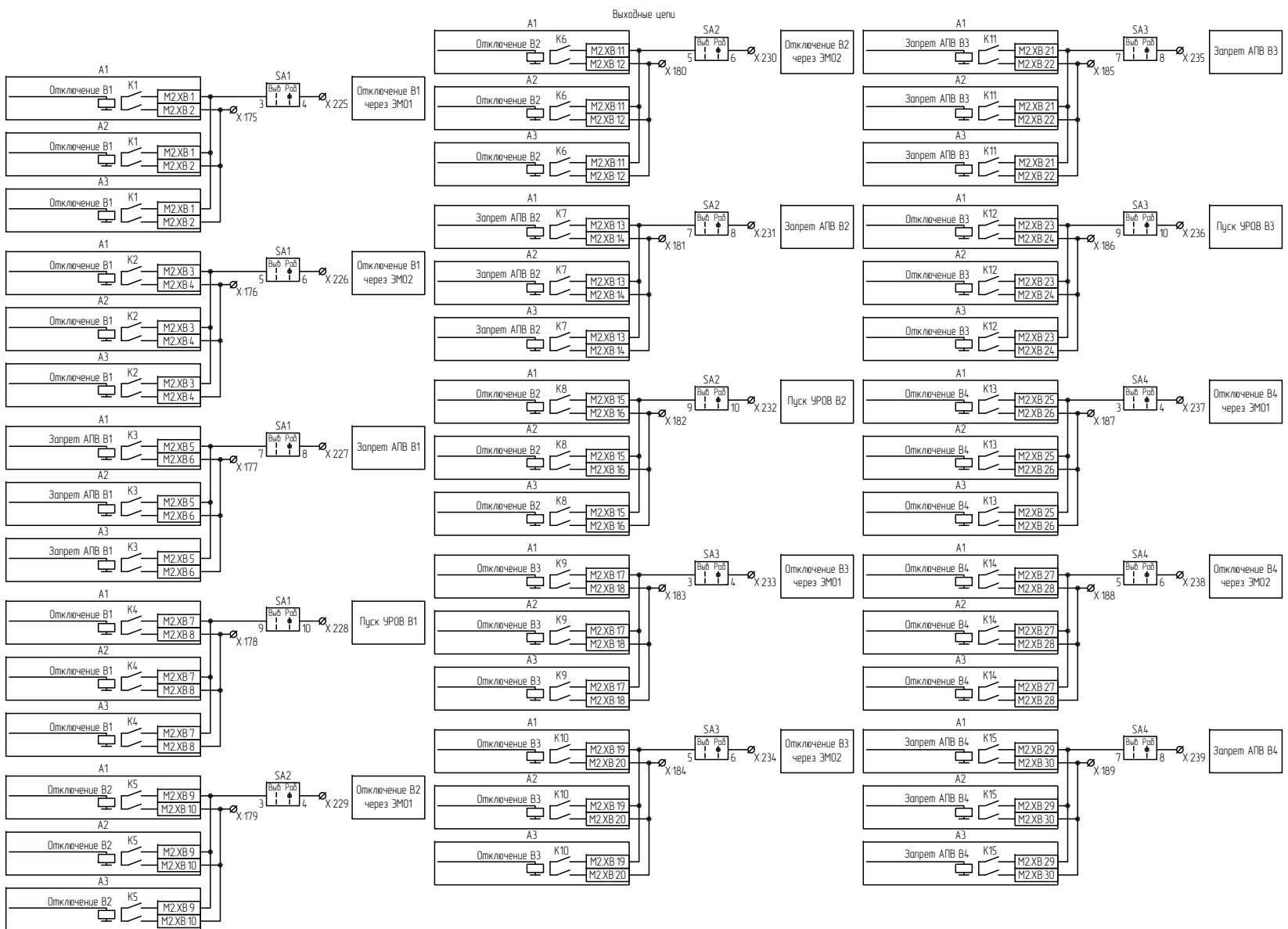
Рисунок Г.8 – Схема электрическая принципиальная (часть 8)
