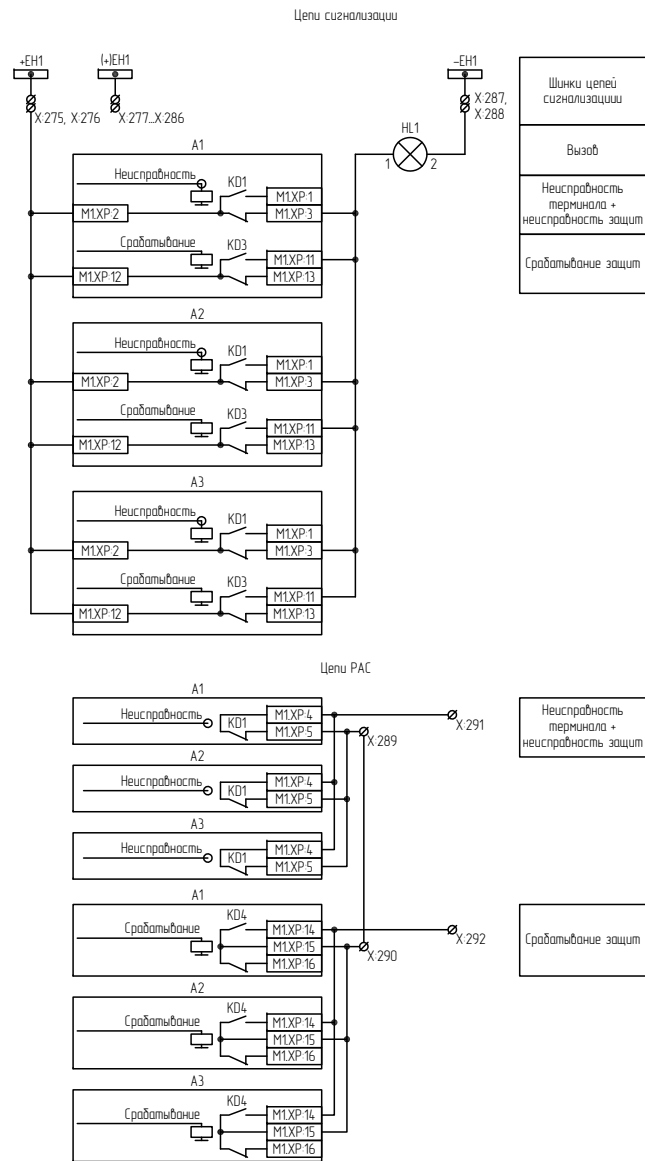
Рисунок Г.11 – Схема электрическая принципиальная (часть 11)
