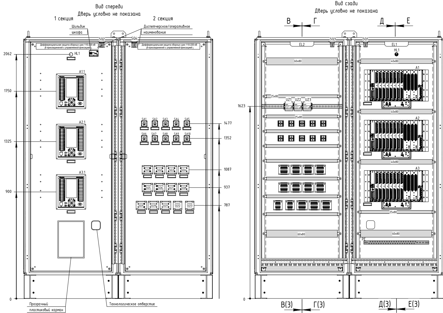
Рисунок В.2 – Чертеж общего вида (часть 2)
